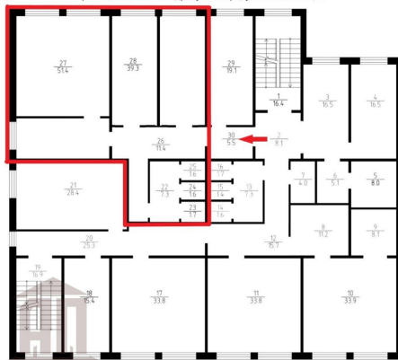
План 3 этажа административно-офисного здания (1-й пусковой комплекс), расположенного по адресу: г. Тверь, ул. Вокзальная, 24
